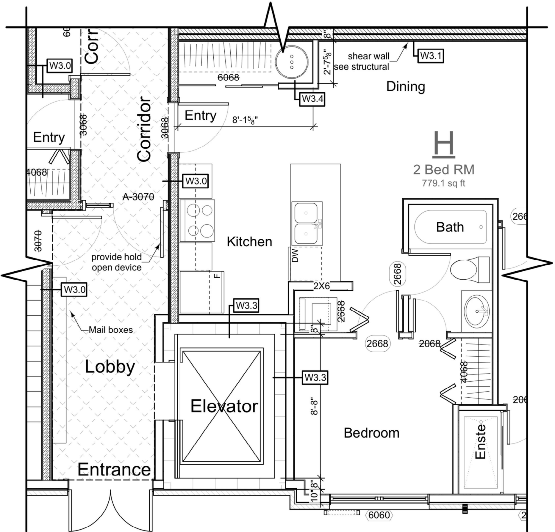
Unit H Layout Scale: 1/4" = 1'-0"
