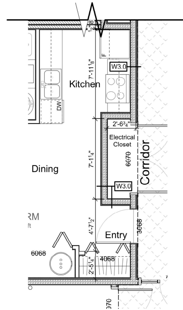
Unit I Layout Scale: 1/4" = 1'-0"
