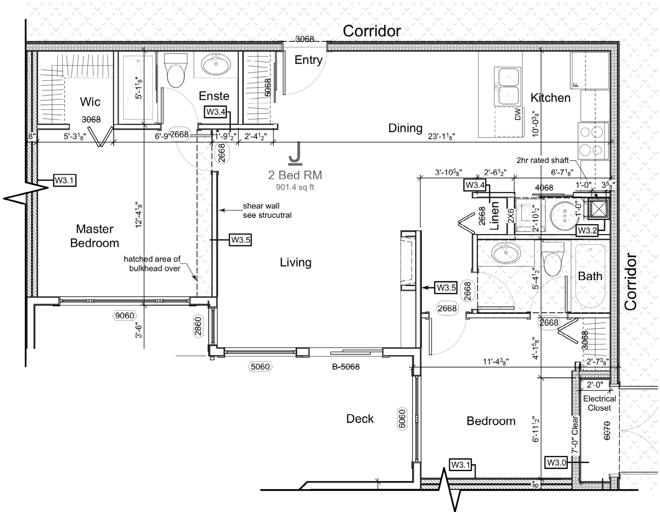
Unit J Layout Scale: 1/4" = 1'-0"
