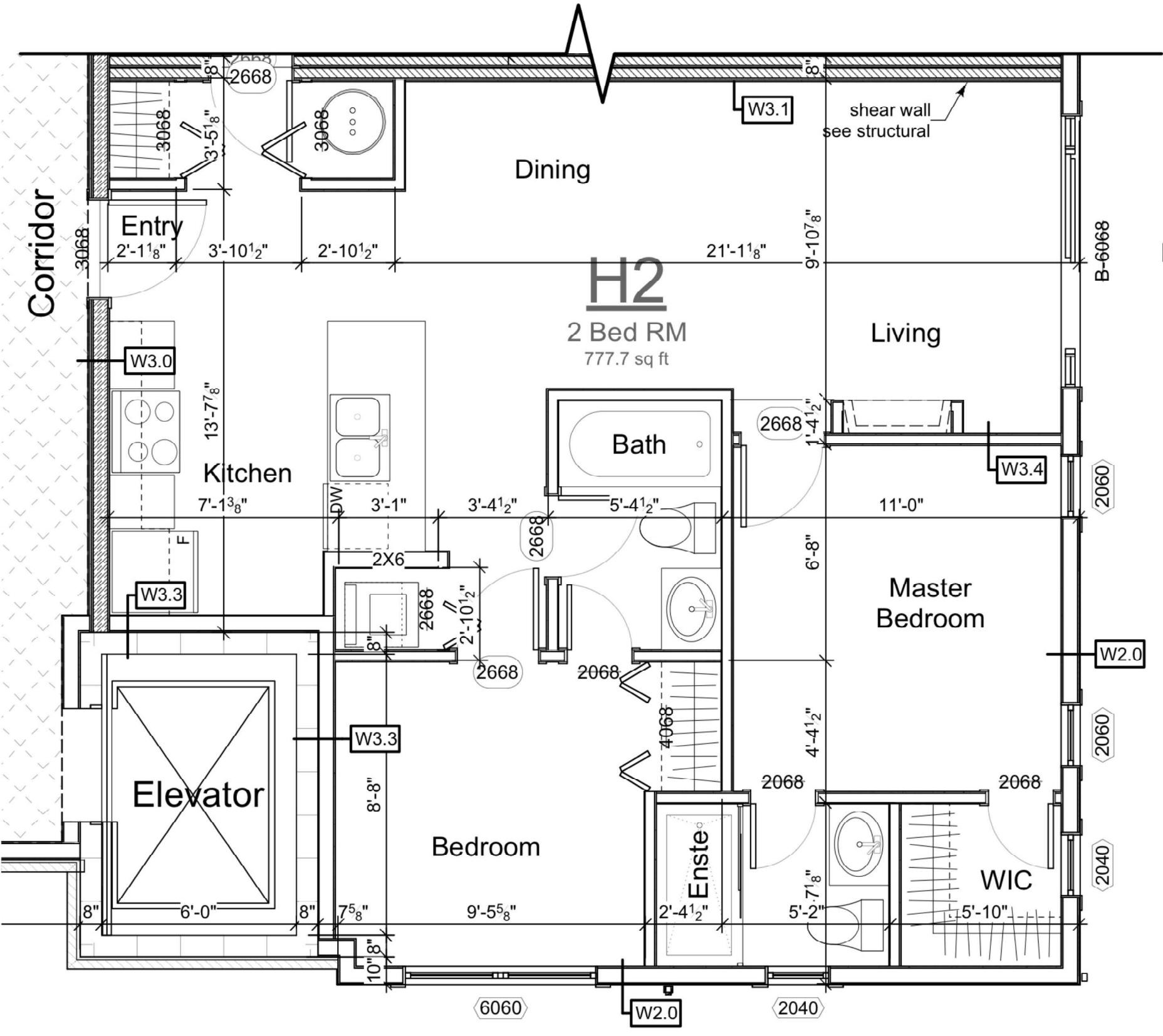
Unit H2 Layout Scale: 1/4" = 1'-0"
