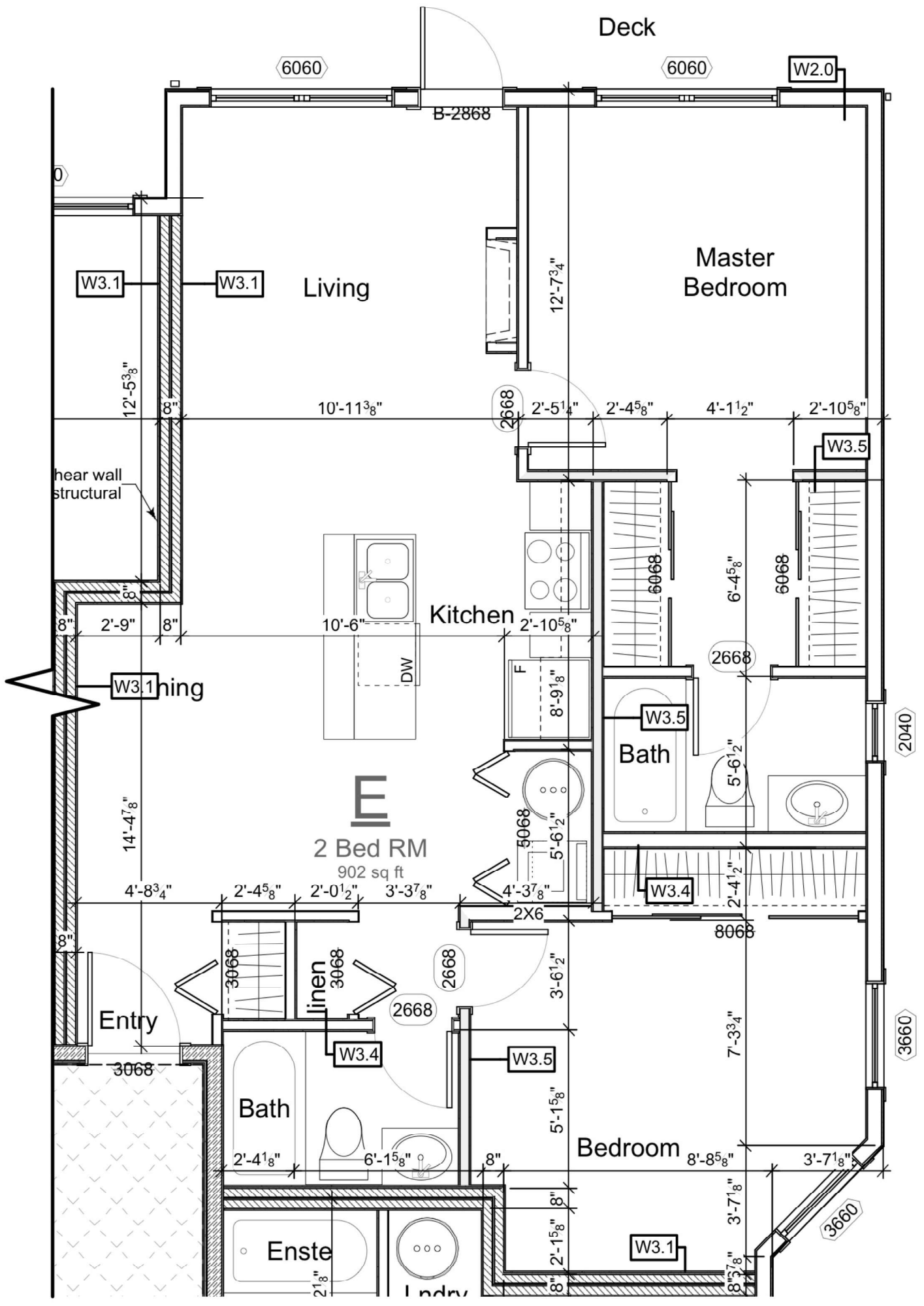
Unit E Layout Scale: 1/4" = 1'-0"
