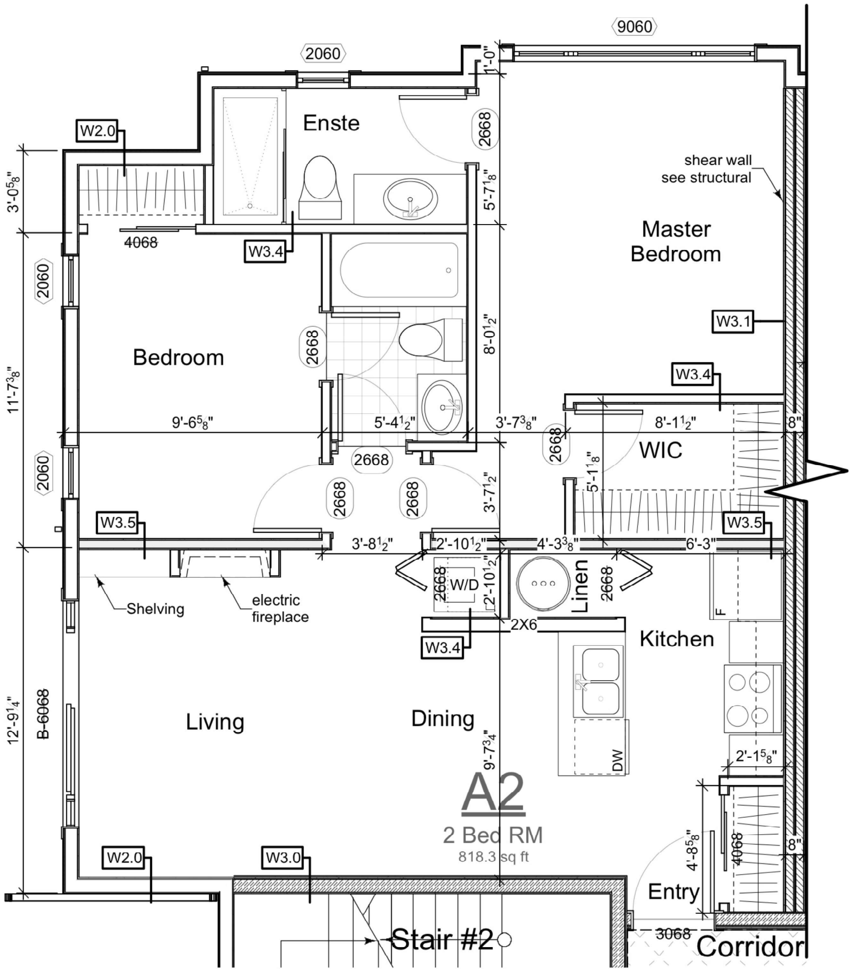
Unit A Layout Scale: 1/4" = 1'-0"
