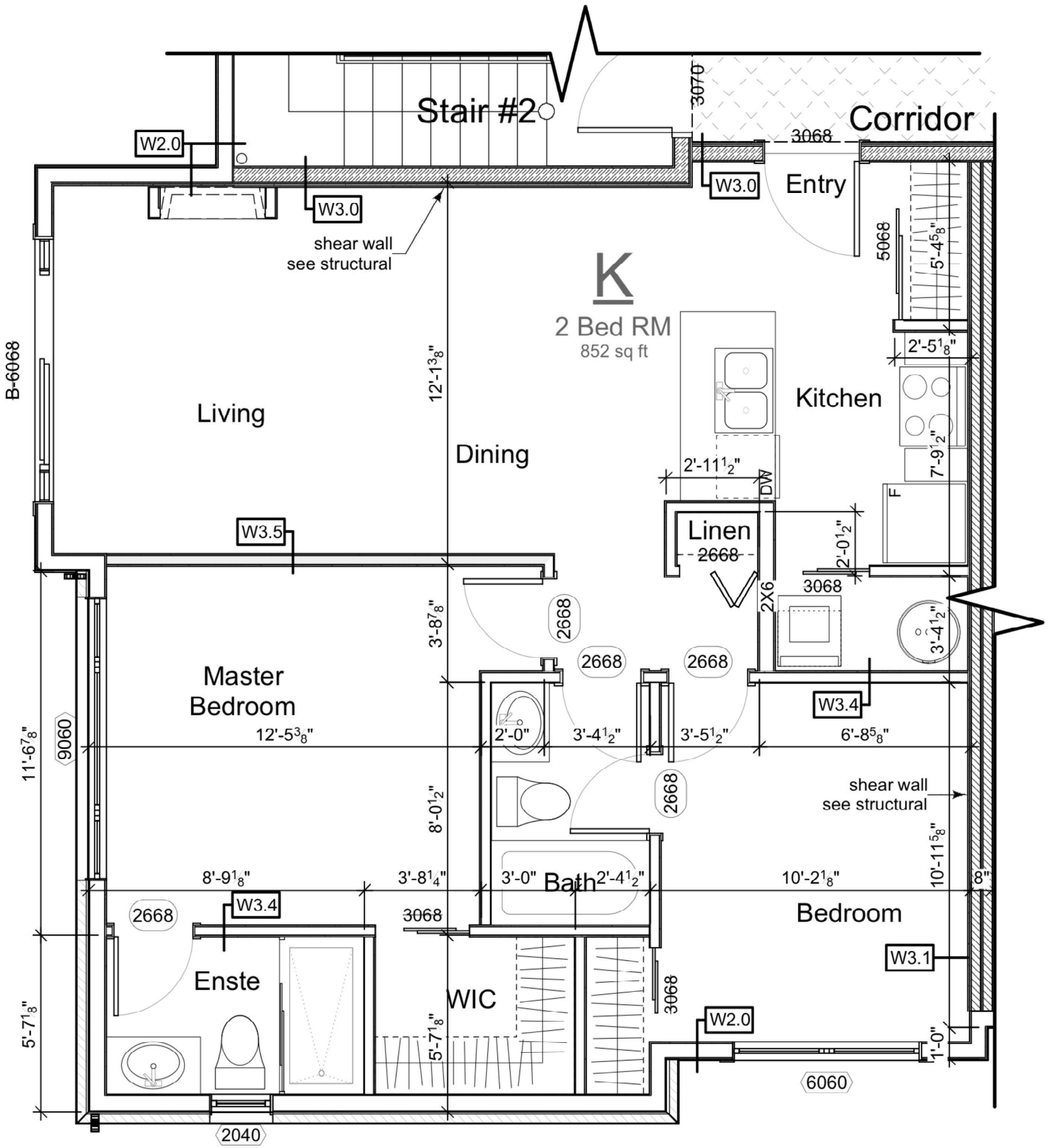
Unit K Layout Scale: 1/4" = 1'-0"
