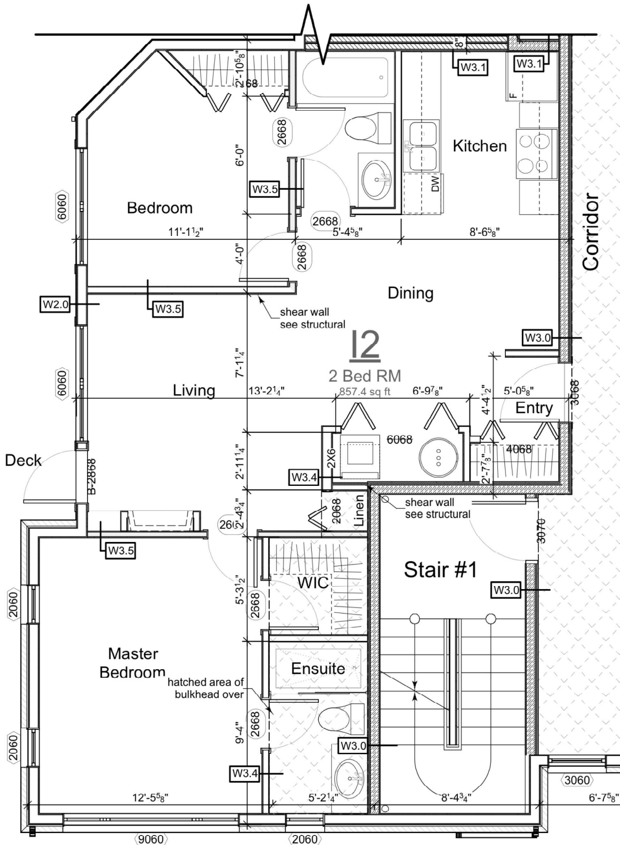
Unit I2 Layout Scale: 1/4" = 1'-0"
